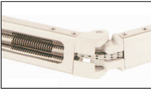
Einblick in den stabilen Kettenarm-Markise der Gelenkarmmarkise >Luxus Sun< .
